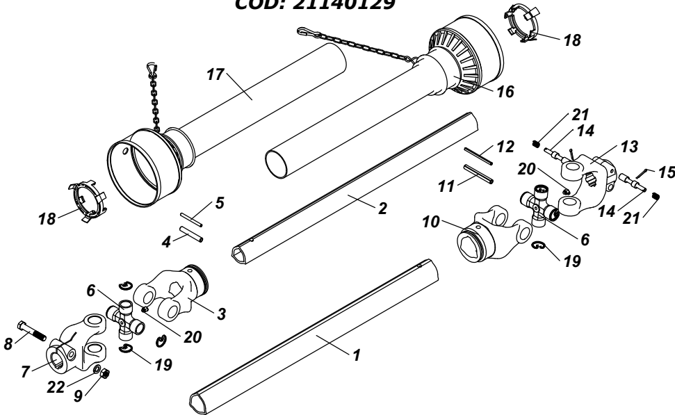
CARDAN KO-41 SÉRIE 007-AENCO 07001125/1190PTT CÓD: 21140129
