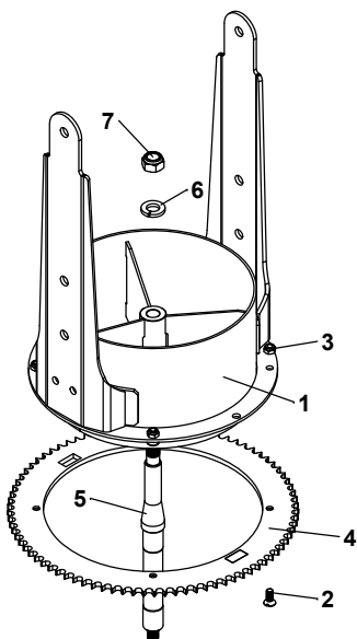
CONDUTOR DIRECIONADOR C/ACIONAMENTO HIDRAULICO COM COROA CÓD: 17395700
