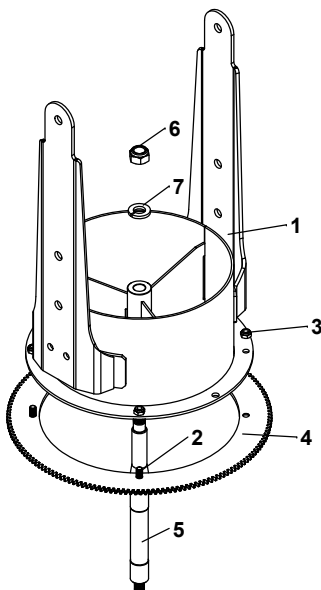
CONDUTOR DIRECIONADOR MOTOR ELETRICO COM COROA CÓD: 17412800
