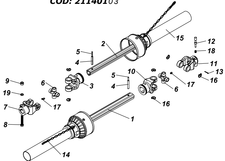
CARDAN KO 32 SERIE 004 COD: 21140103
