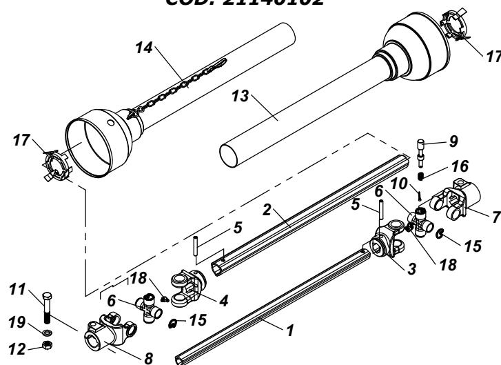
CARDAN KO-31 SERIE 1000(AENCO 01001231/900PT) CÓD: 21140102
