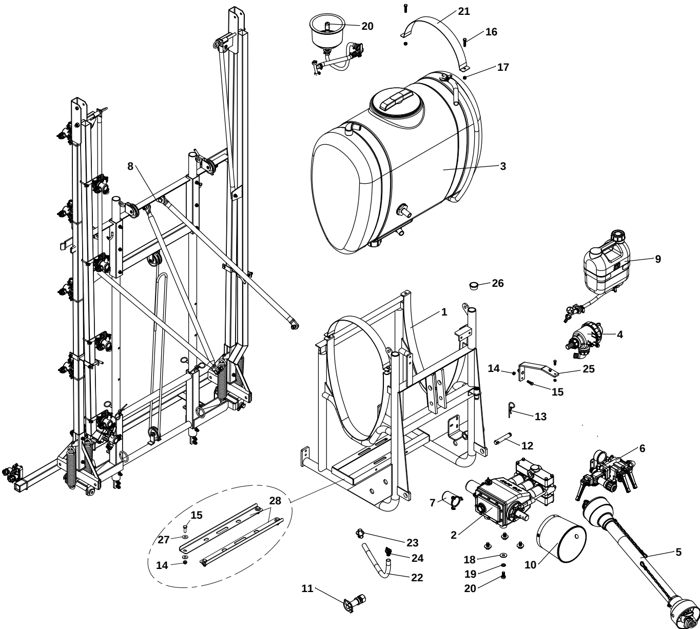
PULVERIZADOR KO 200/300-08/10 (2019)
